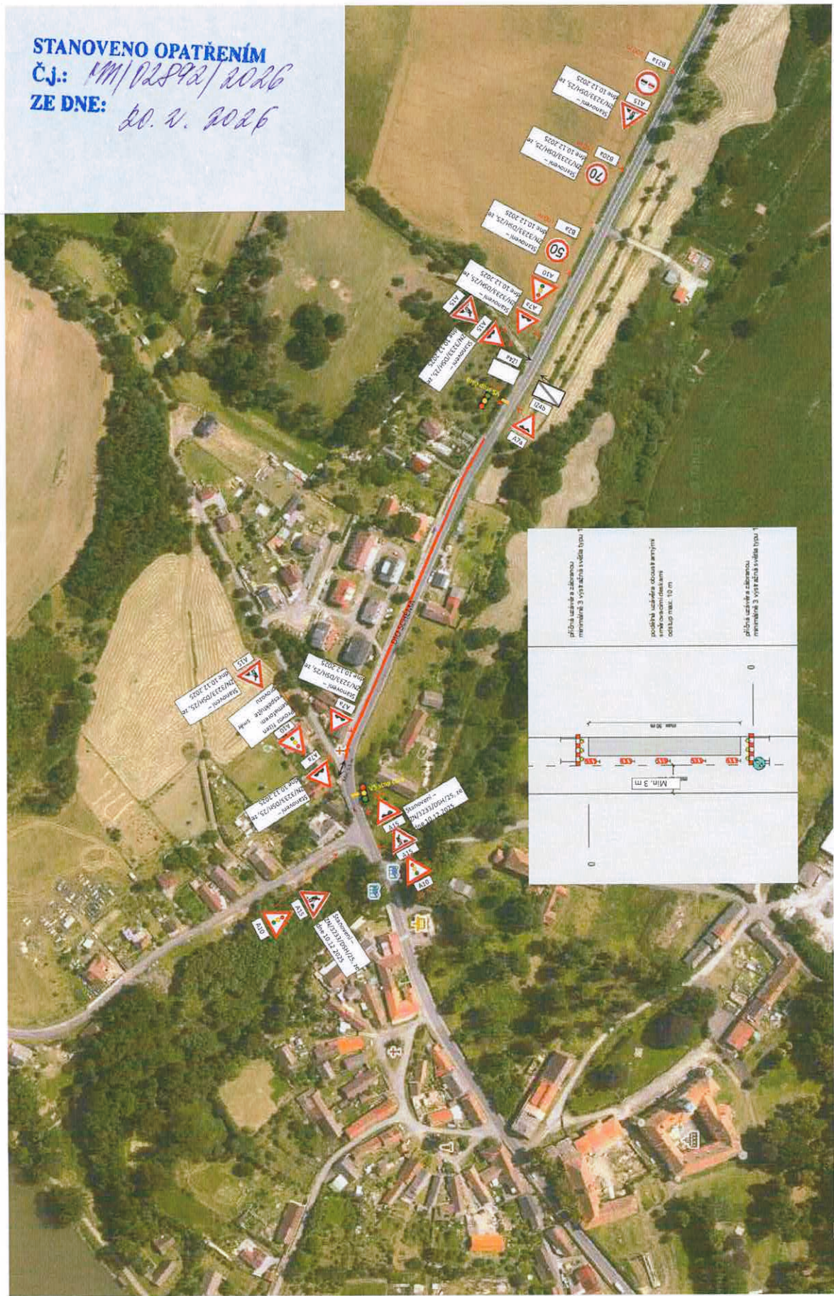
Nalžovské Hory – výměna vodovodu PE63 za PE90 Etapa – I.
